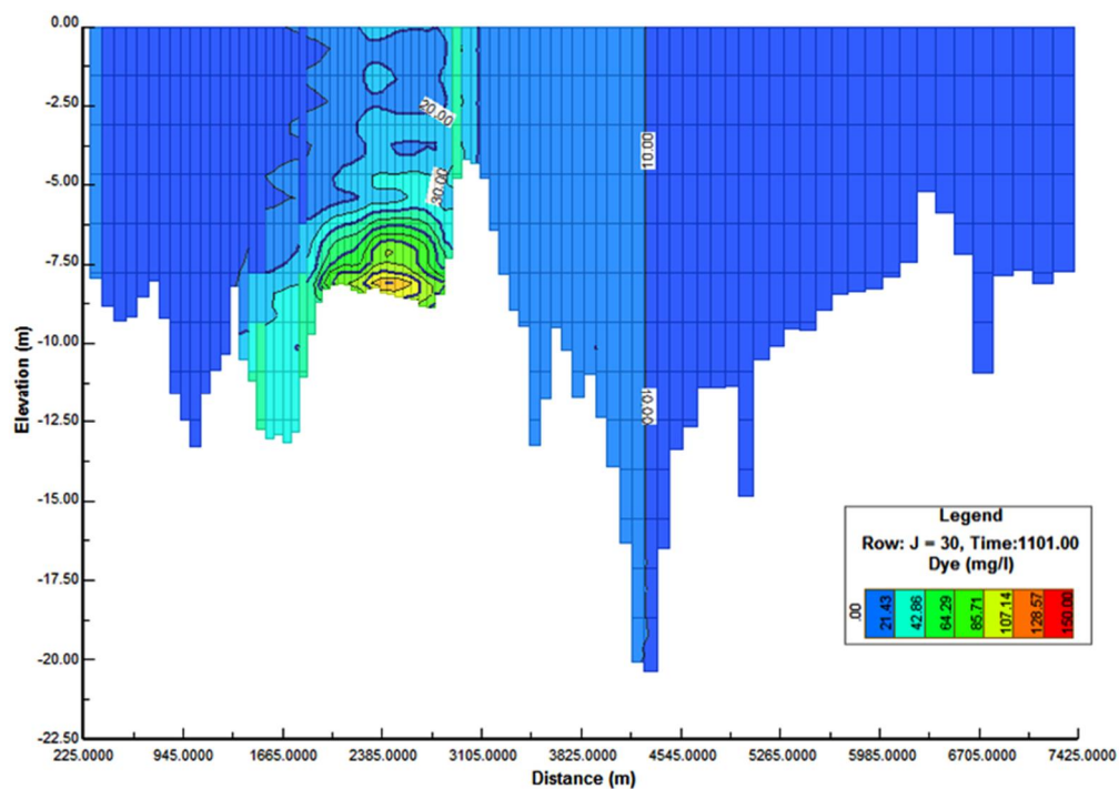
Kuva 8-3. Länsi-itä-suuntainen poikkileikkaus 100 metriä purkuputkesta pohjoiseen. Etelätuuli 5 m/s.
