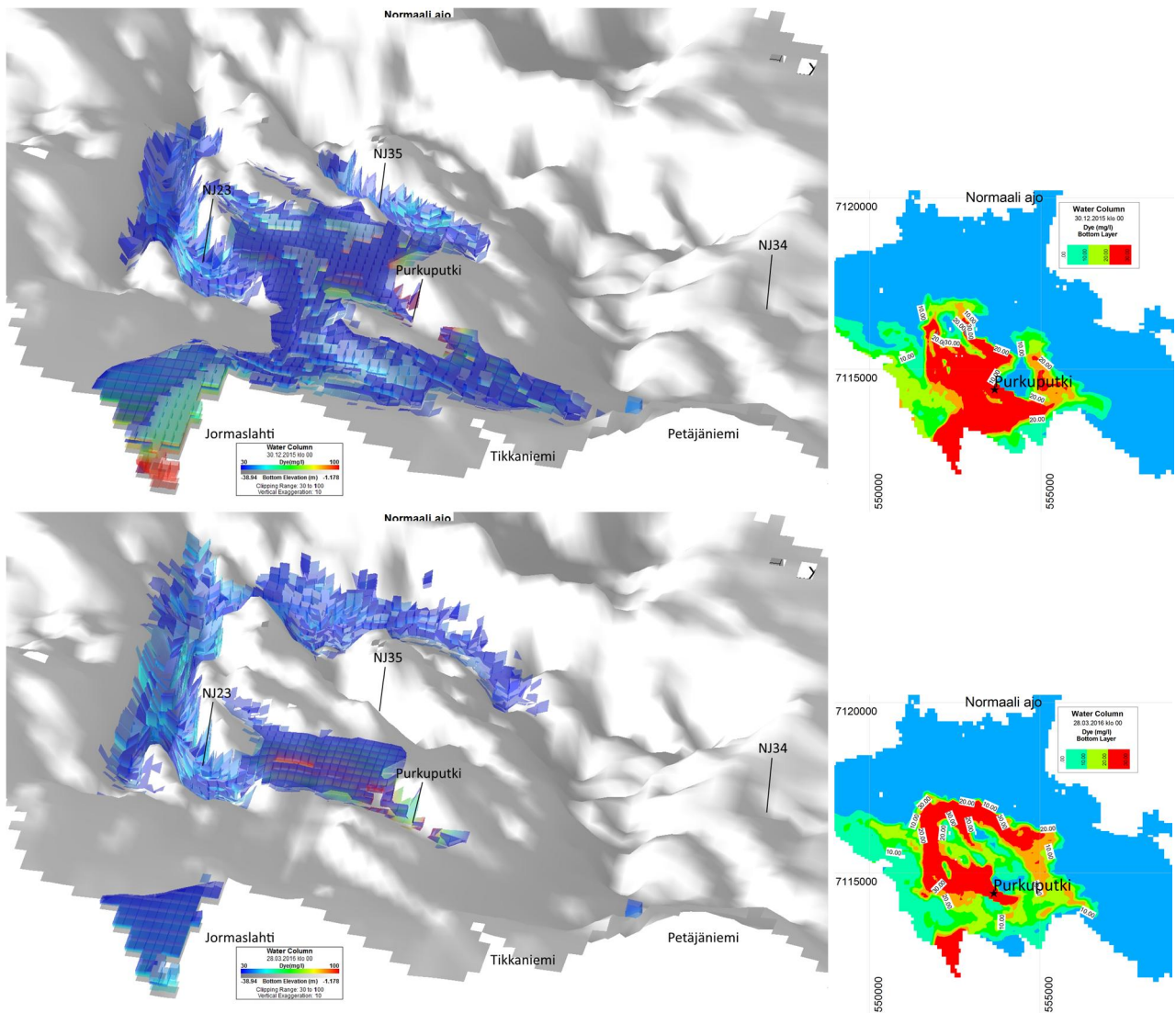
Kuva 8-7. Sulfaattipitoisuus (mg/l) 30.12.2015 ja 28.3.2016 normaalilla Tenetin tulovirtaamalla ja 5 mg/l alkutilan sulfaatilla koko järressä. 3D-kuvissa esitetään vain pitoisuudet välillä 30 – 100 mg/l. Oikeanpuoleisissa pohjakerroksen jakaumakuissa pitoisuusskala on 0 – 30 mg/l. Pisteiden esitetty sijainti on likimääräinen.
