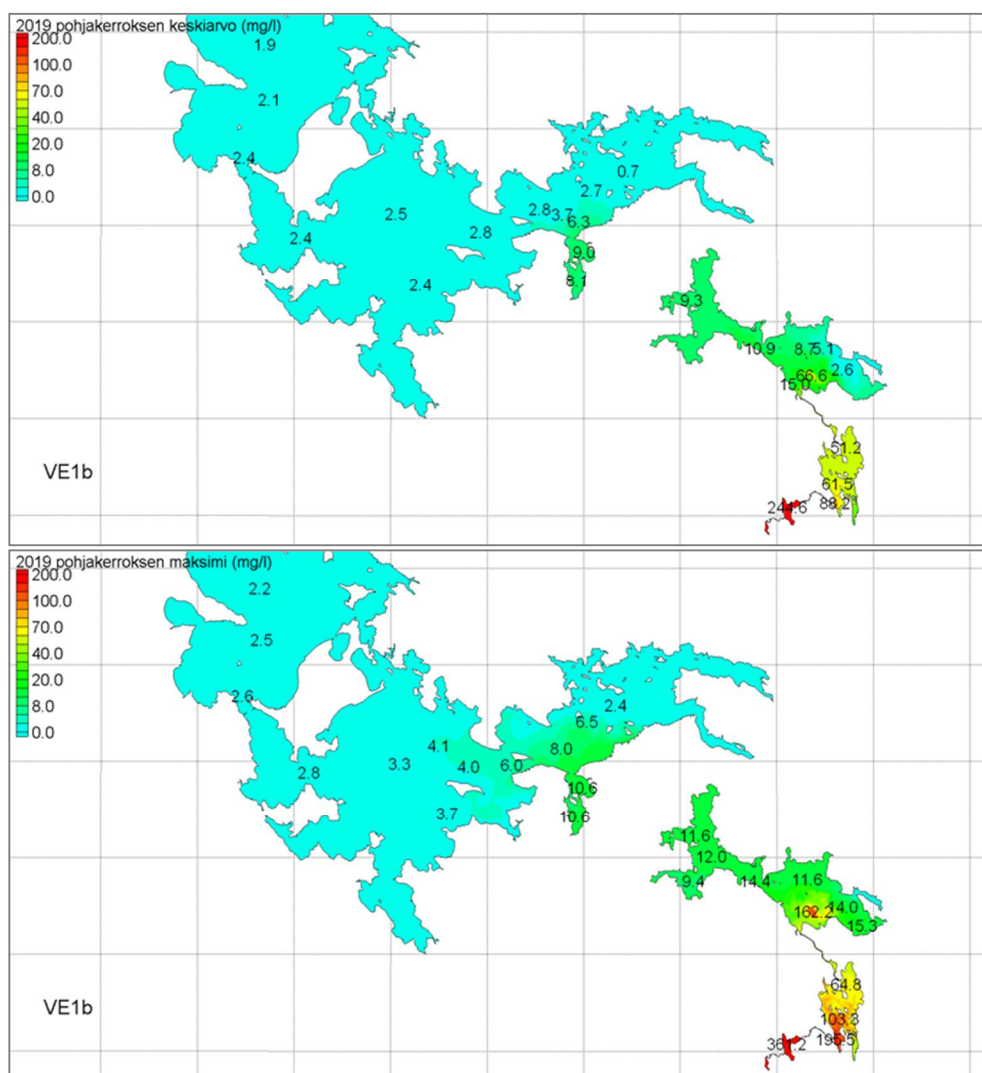
Kuva 5-7. Sulfaattipitoisuuden (mg/l) vuosikeskiarvot ja maksimiarvot 3. laskentavuotena (2019) pohjajärroksessä. Kuormitus Nuasjärven purkuputkeen 15 000 t/v ja Kolmisopen kautta 9 000 t/v. Taustaruudutus 10x10 km. Pohjajärros = mallinnuksen alin vesikerros.
