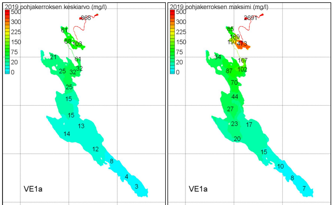
Kuva 5-5. Sulfaattipitoisuuden (mg/l) vuosikeskiarvot ja maksimi-arvot pohjakerroksessa 3. laskentavuotena (2019). Kuormitus Lumijoen kautta 2 000 t/v. Taustaruudutus 5x5 km. Pohjakerros = mallinnuksen alin vesikerros.
