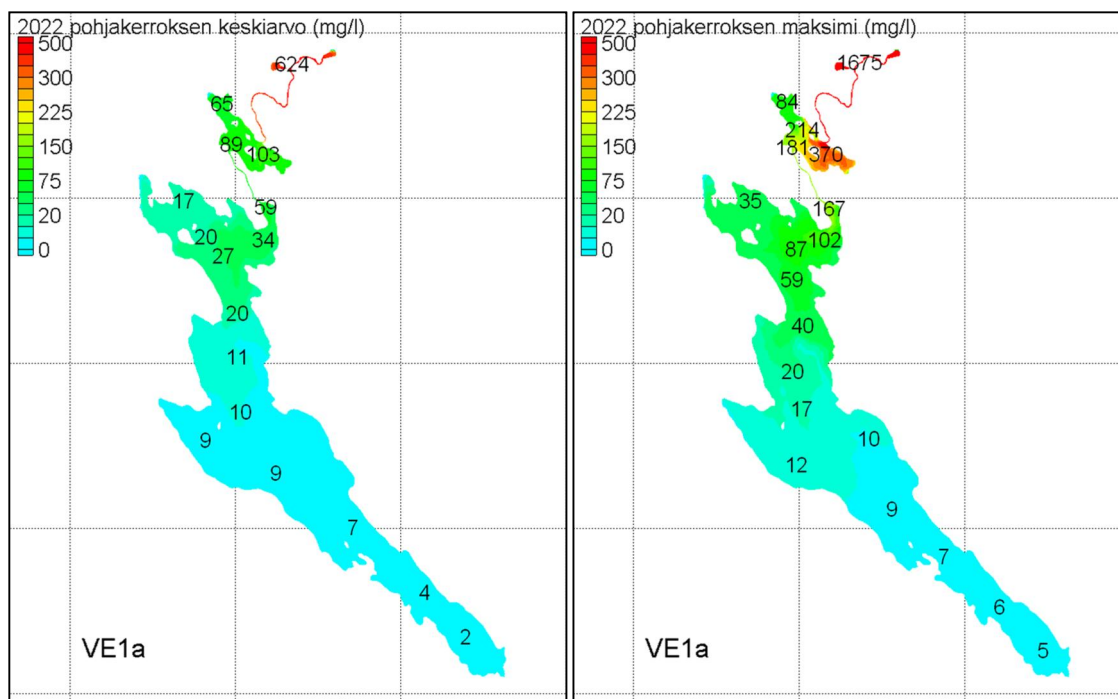
Kuva 5-6. Sulfaattipitoisuuden (mg/l) vuosikeskiarvot ja maksimi-arvot pohjakerroksessa 6. laskentavuotena (2022). Kuormitus Lumijoen kautta 2 000 t/v. Taustaruudutus 5x5 km. Pohjakerros = mallinnuksen alin vesikerros.
