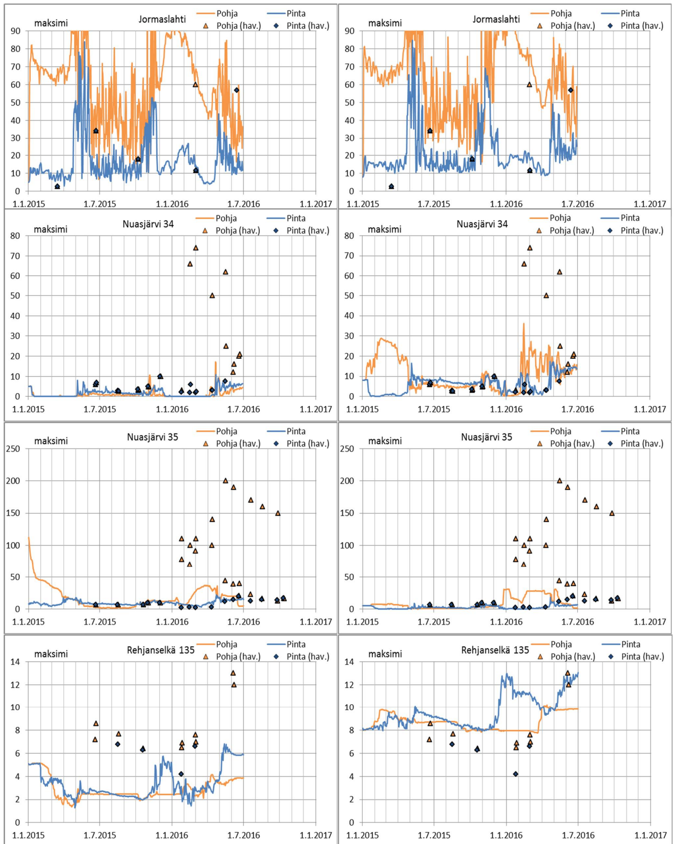
Kuva 8-5. Sulfaattipitoisuuden (mg/l) vaihtelu pinnassa ja pohjassa Nuasjärven tarkennetun hilan malliajossa (vasemmanpuoleiset kuvat) vs. tilanne, jossa Tenetin virtaama on pudotettu kolmasosaan (oikeanpuoleiset kuvat). Tarkastelupisteiden sijainti on esitetty kuvissa (Kuva 8-4 ja Kuva 3-4).
