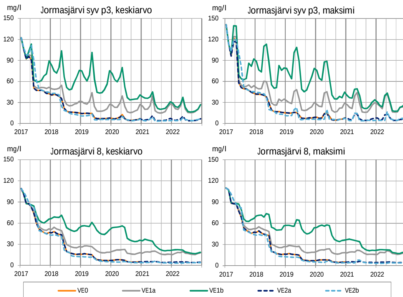
Kuva 6-1. Sulfaattipitoisuuden (mg/l) keskimääräinen vaihtelu Jormasjärvessä pohjakerroksessa eri vaihtoehtoissa. Pohjakerros = mallinnuksen alin vesikerros.
