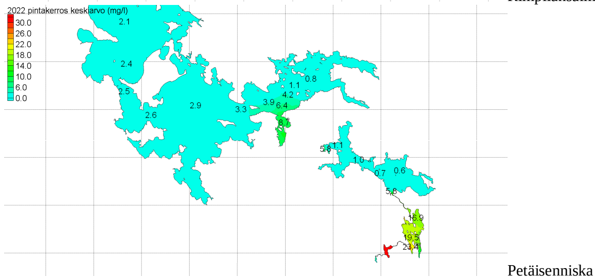
Kuva 4-8. Sulfaattipitoisuuden keskiarvot pintakerroksessa 6. vuotena (2022) kuivana vesivuotena Nussjärven purkutupken kuormituksen ollessa 15 000 tn/v (VE1a) eri purkupaikkavaihtoehtoissa. Taustaruudutus 10x10 km. Pintakerros = mallinnuksen ylin vesikerros.
