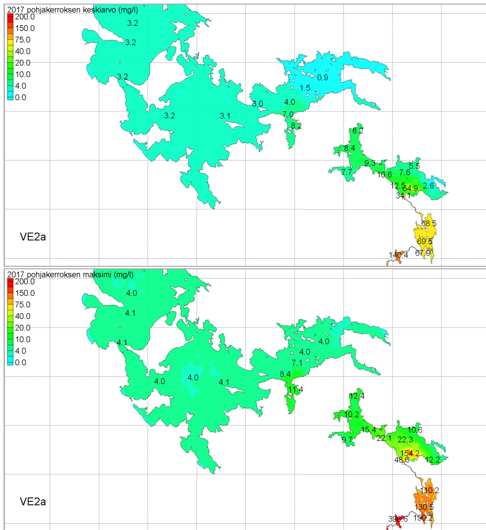
Kuva 5-11. Sulfaattipitoisuuden (mg/l) vuosikeskiarvot ja maksimiarvot pohjakerroksessa 1. laskentavuotena (2017). Kuormitus Nuasjärven purkuputkeen 16 000 t/v ja Kolmisopen kautta noin 840 t/v. Taustaruudutus 10x10 km. Pohjakerros = mallinnuksen alin vesikerros.
