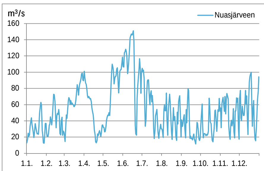
Kuva 3-1. Mallinnuksessa käytetty Nuasjärveen tuleva virtaama.
