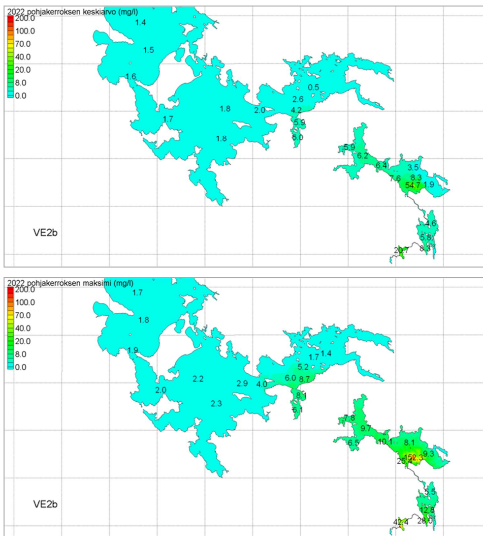
Kuva 5-14. Sulfaattipitoisuuden (mg/l) vuosikeskiarvot ja maksimi-arvot pohjakerroksessa 6. laskentavuotena (2022). Kuormitus Nuasjärven purkuputkeen 11 800 t/v ja Kolmisopen kautta noin 840 t/v. Taustaruudutus 10x10 km. Pohjakerros = mallinnuksen alin vesikerros.
