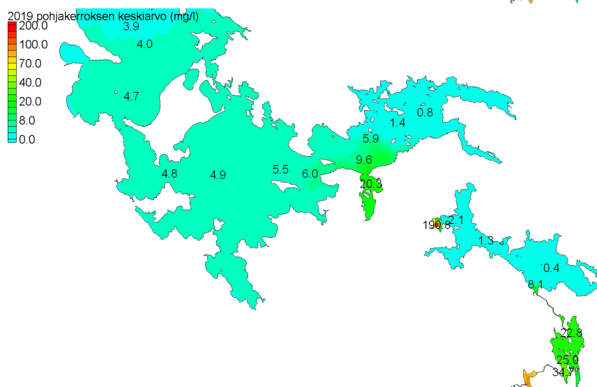
Kuva 4-6. Sulfaattipitoisuuden keskiarvot pohjakerroksessa 3. vuotena (2019) kuivana vesivuotena Nuasjärven purkuputken kuormituksen ollessa 30 000 tn/v (VE1a) eri purkupaikkavaihtoehdoissa. Pohjakerros = mallinnuksen alin vesikerros.
