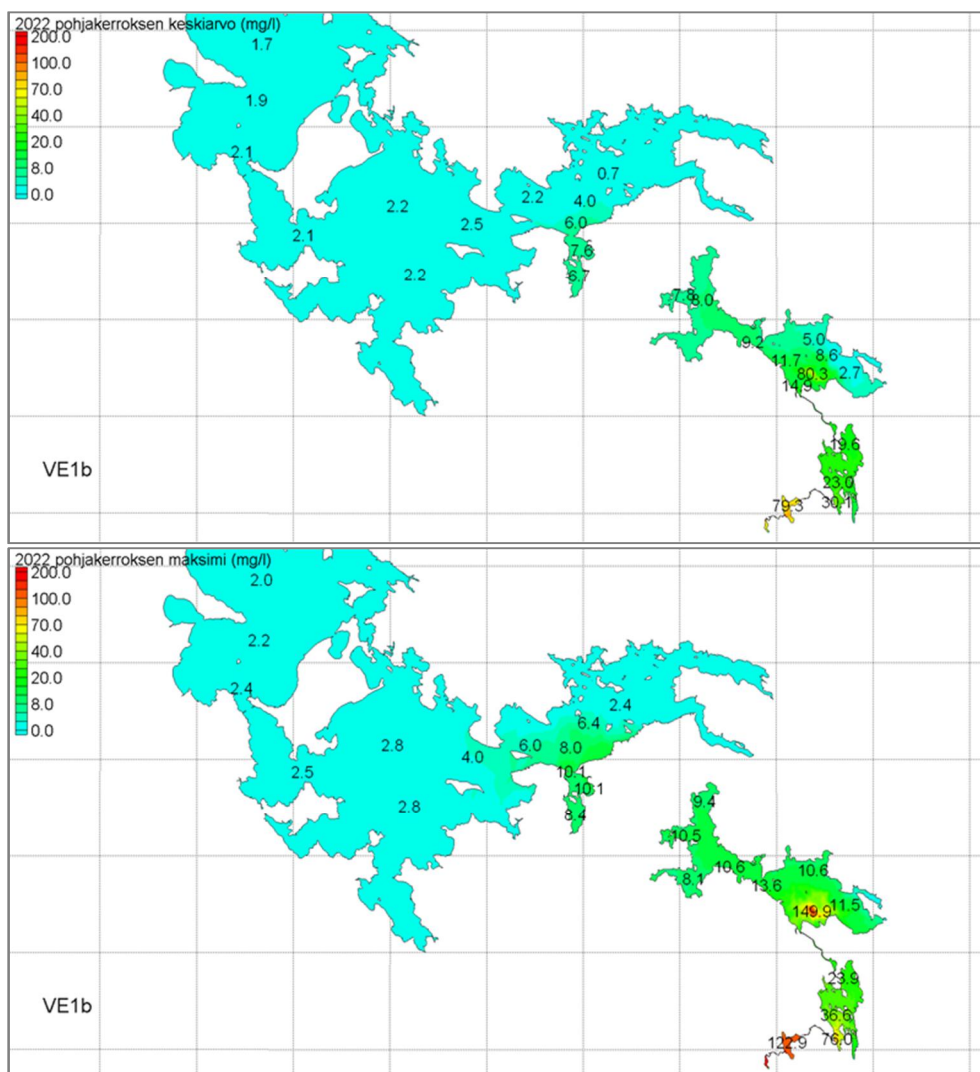
Kuva 5-8. Sulfaattipitoisuuden (mg/l) vuosikeskiarvot ja maksimi-arvot pohjakerroksessa 6. laskentavuotena (2022). Kuormitus Nuasjärven purkuputkeen 15 000 t/v ja Kolmisopen kautta 3 000 t/v. Taustaruudutus 10x10 km. Pohjakerros = mallinnuksen alin vesikerros.
