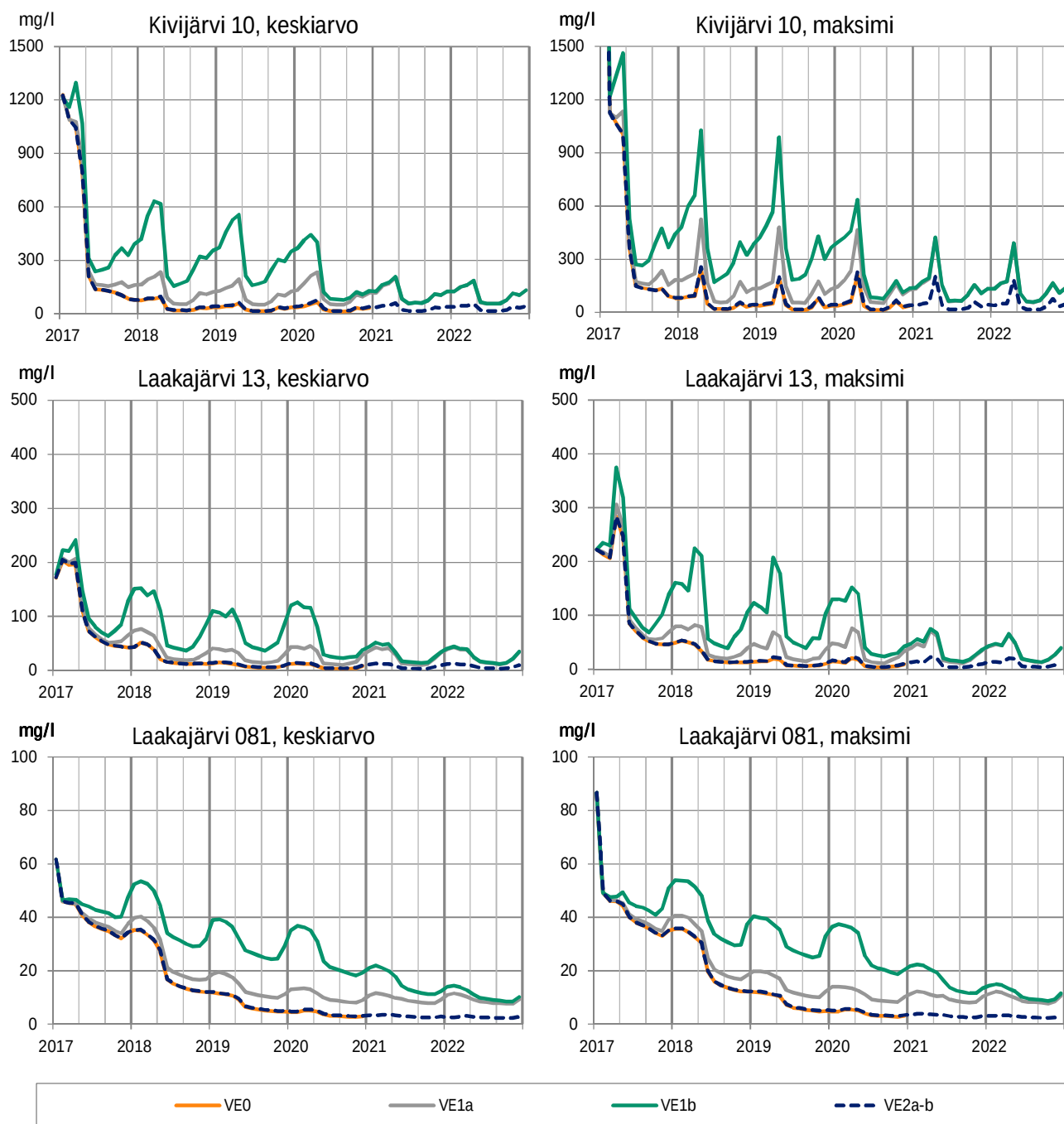
Kuva 6-2. Sulfaattipitoisuuden (mg/l) keskimääräinen vaihtelu Kivijärvässä ja Laakajärvässä pohjakerroksessa eri vaihtoehtoissa. Pohjakerros = mallinnuksen alin vesikerros.
