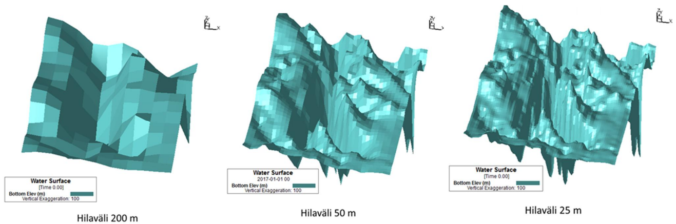
Kuva 3-3. Nuasjärven purkupaikan lähiympäristön syvänealue hilakooalla 200 m, 50 m ja 25 m.
