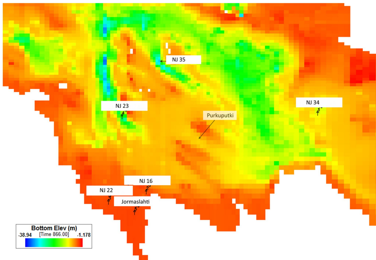
Kuva 8-4. Nuasjärven tarkennettun mallinnusalueen syvyysuhteet ja tarkastelupisteet.
