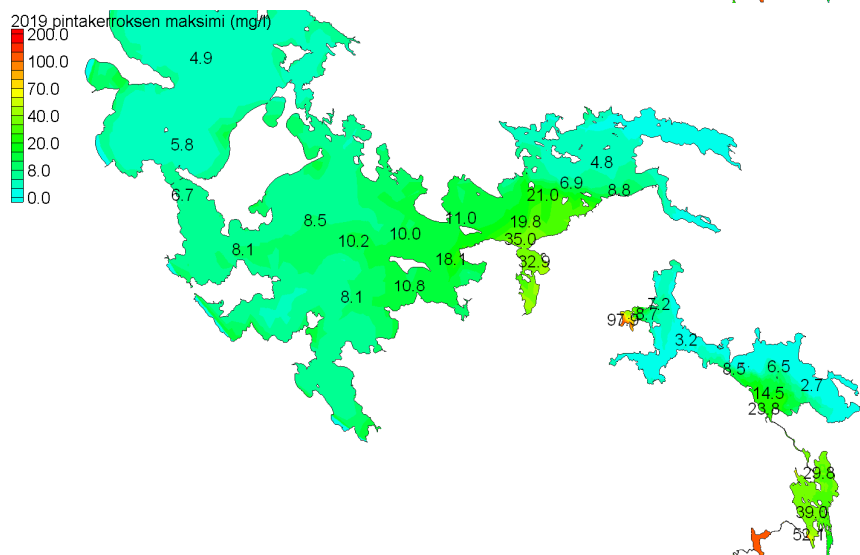
Kuva 4-5. Sulfaattipitoisuuden vuosimaksimit pintakerroksessa 3. vuotena (2019) kuivana vesivuotena Nuasjärven purkupuolen kuormituksen ollessa 30 000 tn/v (VE1a) eri purkupaikkavaihtoehtoissa: nykyinen, Rimpilänsalmi ja Petäisenniska. Pintakerros = mallinnuksen ylin vesikerros.
