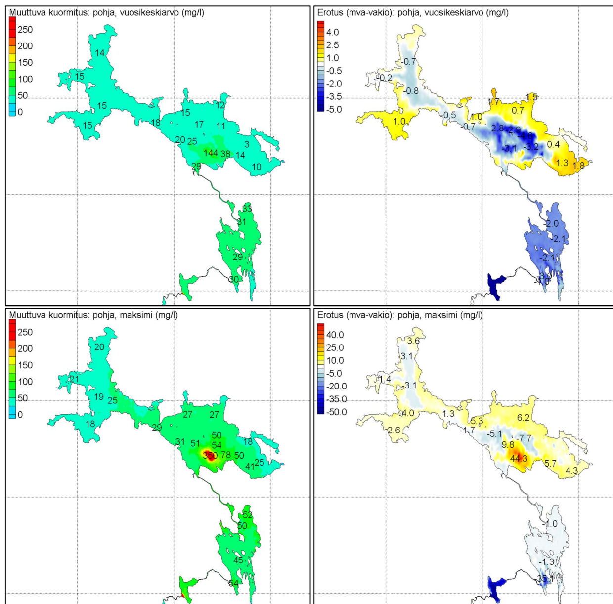
Kuva 7-1. Sulfaattipitoisuuden (mg/l) vuosikeskiarvot ja maksimit pohjakerroksessa 2. laskentavuotena (2018), kuormitus (Nuasjärven purkuputki 30 000 t/v ja Kolmisopen kautta 3000 t/v) jaksoitettuna vuodenajan mukaan. Oikean puoleisissa jakaumakuviissa on esitetty keskimääräinen pitoisuusero jaksotetun ja tasaisen kuormituksen jakaumien välillä. Pohjakerros = mallinnuksen alin vesikerros
