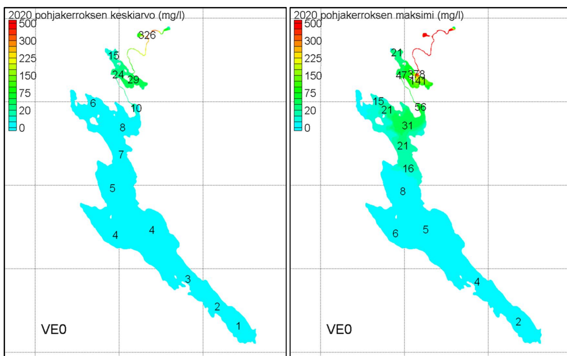
Kuva 5-2. Sulfaattipitoisuuden (mg/l) vuosikeskiarvot ja maksimiarvot pohjakerroksessa 4. laskentavuotena (2020). Kuormitus Lumijoen kautta 520 t/v. Taustaruudutus 5x5 km. Pohjakerros = mallinnuksen alin vesikerros.
