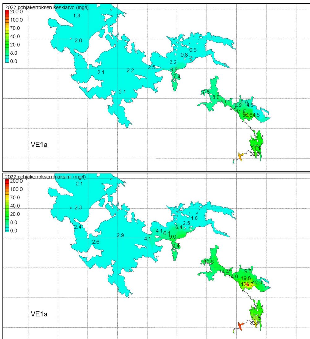
Kuva 5-4. Sulfaattipitoisuuden (mg/l) vuosikeskiarvot ja maksimi-arvot pohjakerroksessa 6. laskentavuotena (2022). Nuasjärven purkupaikan kuormitus 15 000 t/v ja Kolmisopen kautta 3 000 t/v. Taustaruudutus 10x10 km. Pohjakerros = mallinnuksen alin vesikerros.
