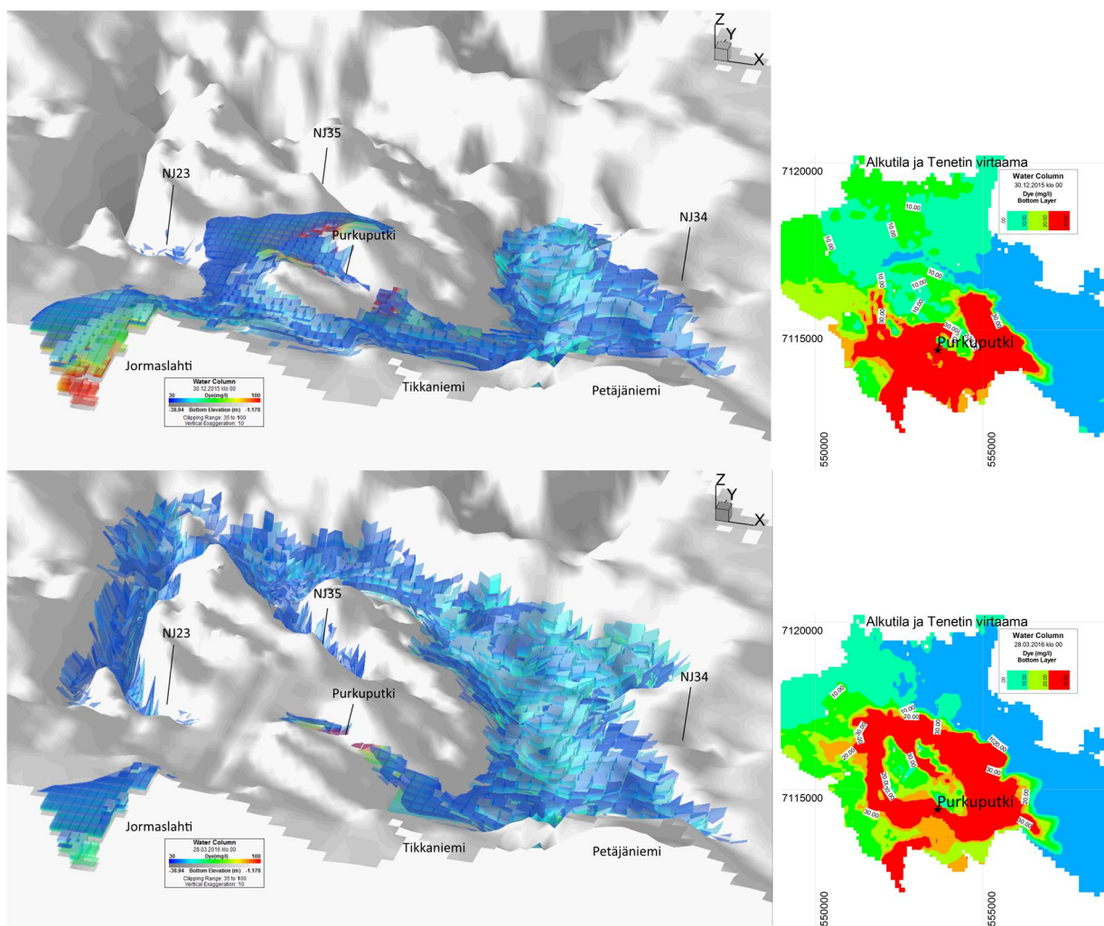
Kuva 8-8. Sulfaattipitoisuus 30.12.2015 ja 28.3.2016 pienennetyllä Tenetin tulovirtaamalla ja korotetulla alkutilan sulfaatilla syvänteissä. 3D-kuvissa esitetään vain pitoisuudet välillä 30 – 100 mg/l. Oikeanpuoleisissa pohjakerroksen jakaumakuvissa pitoisuusskaala on 0 – 30 mg/l. Pisteiden esitetty sijainti on likimääräinen.
