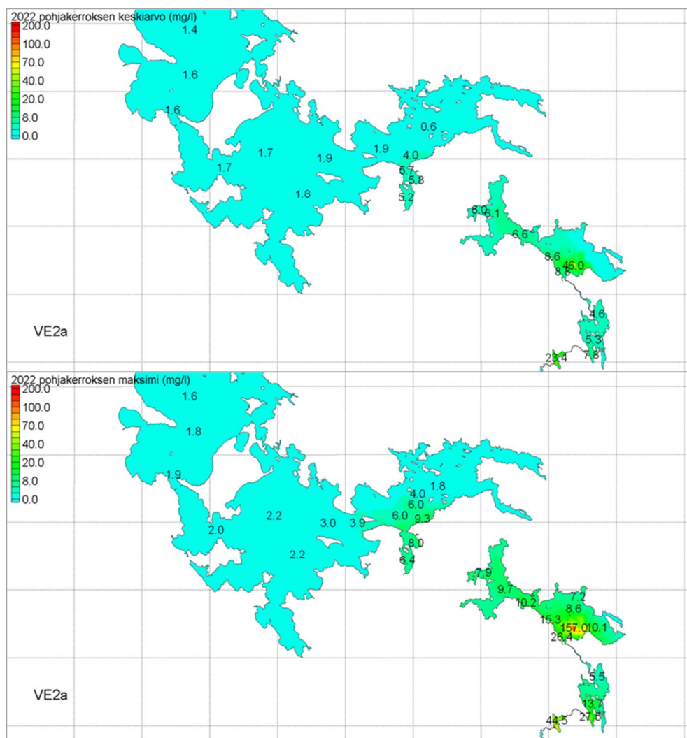
Kuva 5-12. Sulfaattipitoisuuden (mg/l) vuosikeskiarvot ja maksimiarvot pohjakerroksessa 6. laskentavuotena (2022). Kuormitus Nuasjärven purkuputkeen 11 800 t/v ja Kolmisopen kautta noin 840 t/v. Taustaruudutus 10x10 km 2 . Pohjakerros = mallinnuksen alin vesikerros.
