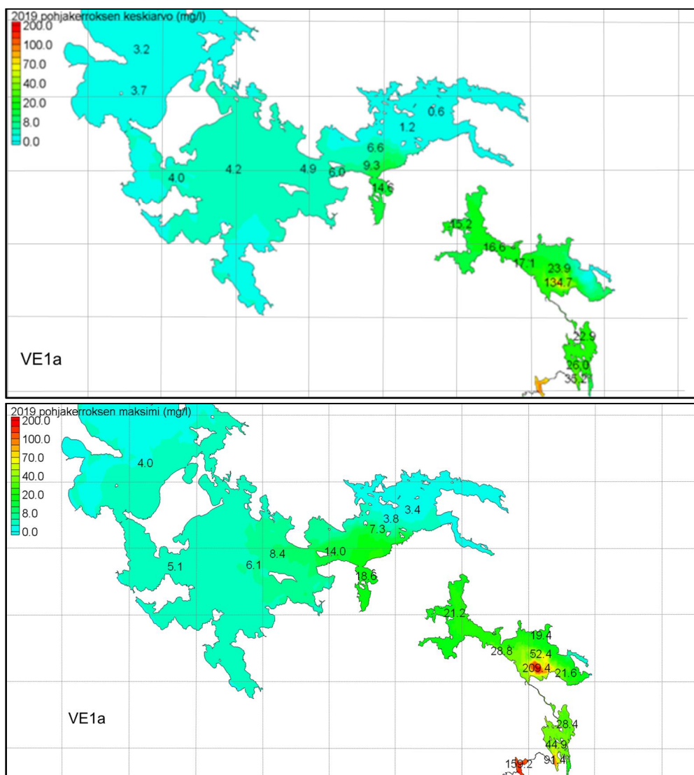
Kuva 5-3. Sulfaattipitoisuuden (mg/l) vuosikeskiarvot ja maksimiarvot pohjakerroksessa 3. laskentavuotena (2019). Nuasjärven purkuputken kuormitus 30 000 t/v ja Kolmisopen kautta 3 000 t/v. Taustaruudutus 10x10 km. Pohjakerros = mallinnuksen alin vesikerros.
