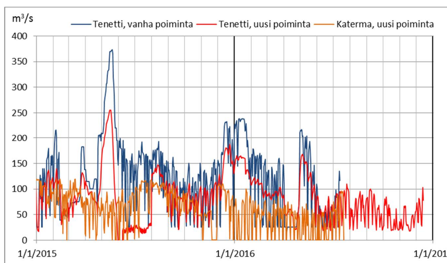
Kuva 8-9. Mallinnuksessa käytetty virtaama ( \text{m}^3/\text{s} ) Tenetissä sinisellä. Punaisella pienempi virtaama, poiminta tehty myöhemmin. Lisäksi oranssilla on esitetty juoksutukset ylempänä Katerman kohdalla.
