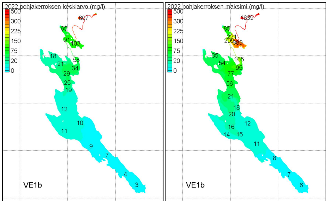
Kuva 5-10. Sulfaattipitoisuuden (mg/l) vuosikeskiarvot ja maksimiarvot pohjakerroksessa 6. laskentavuotena (2022). Kuormitus Lumijoen kautta 2 000 t/v. Taustaruudutus 5x5 km. Pohjakerros = mallinnuksen alin vesikerros.
