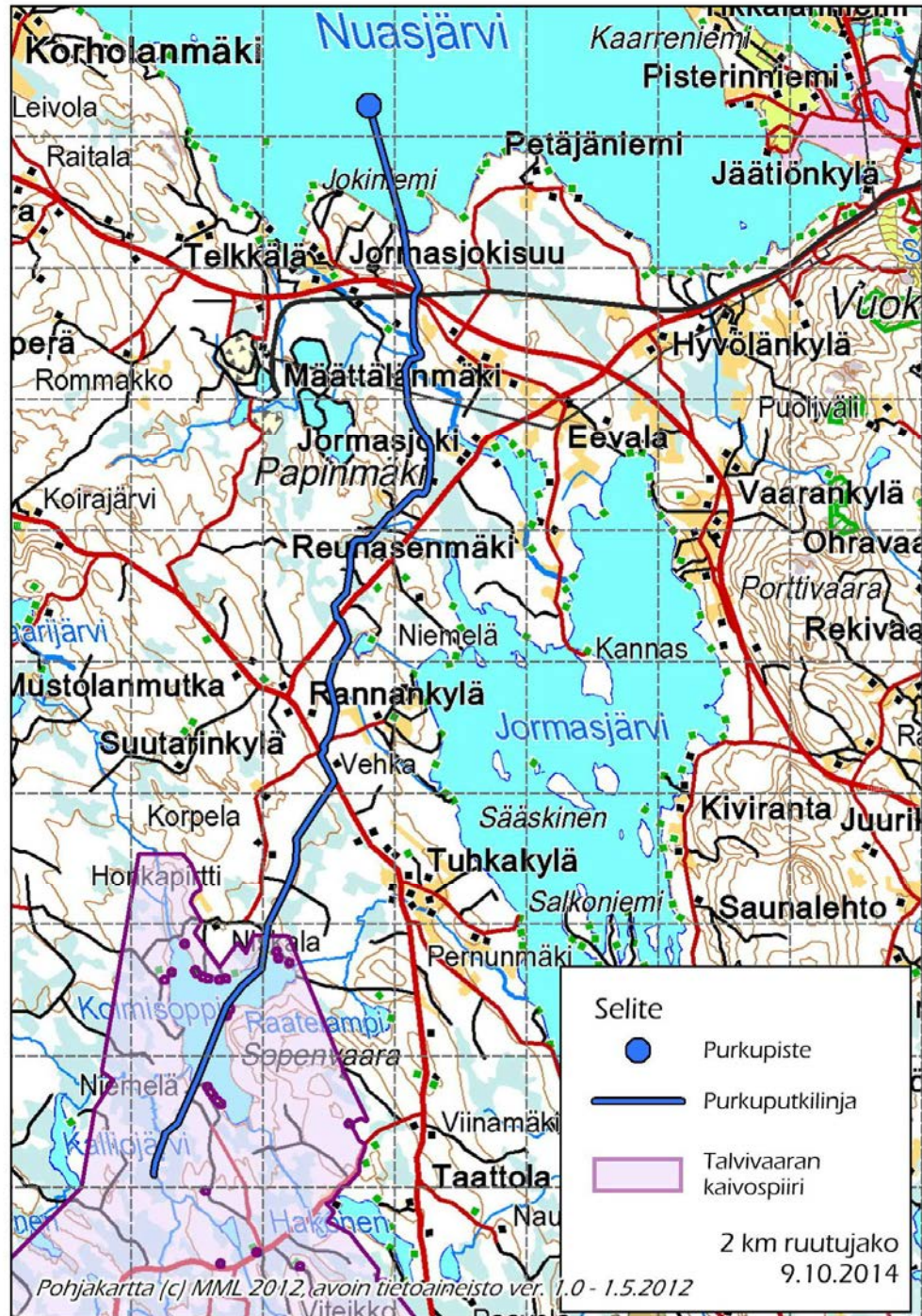
Kuva 4-7. Terrafamen purkuputken linjaus kaivosalueelta Nuasjärveen.
