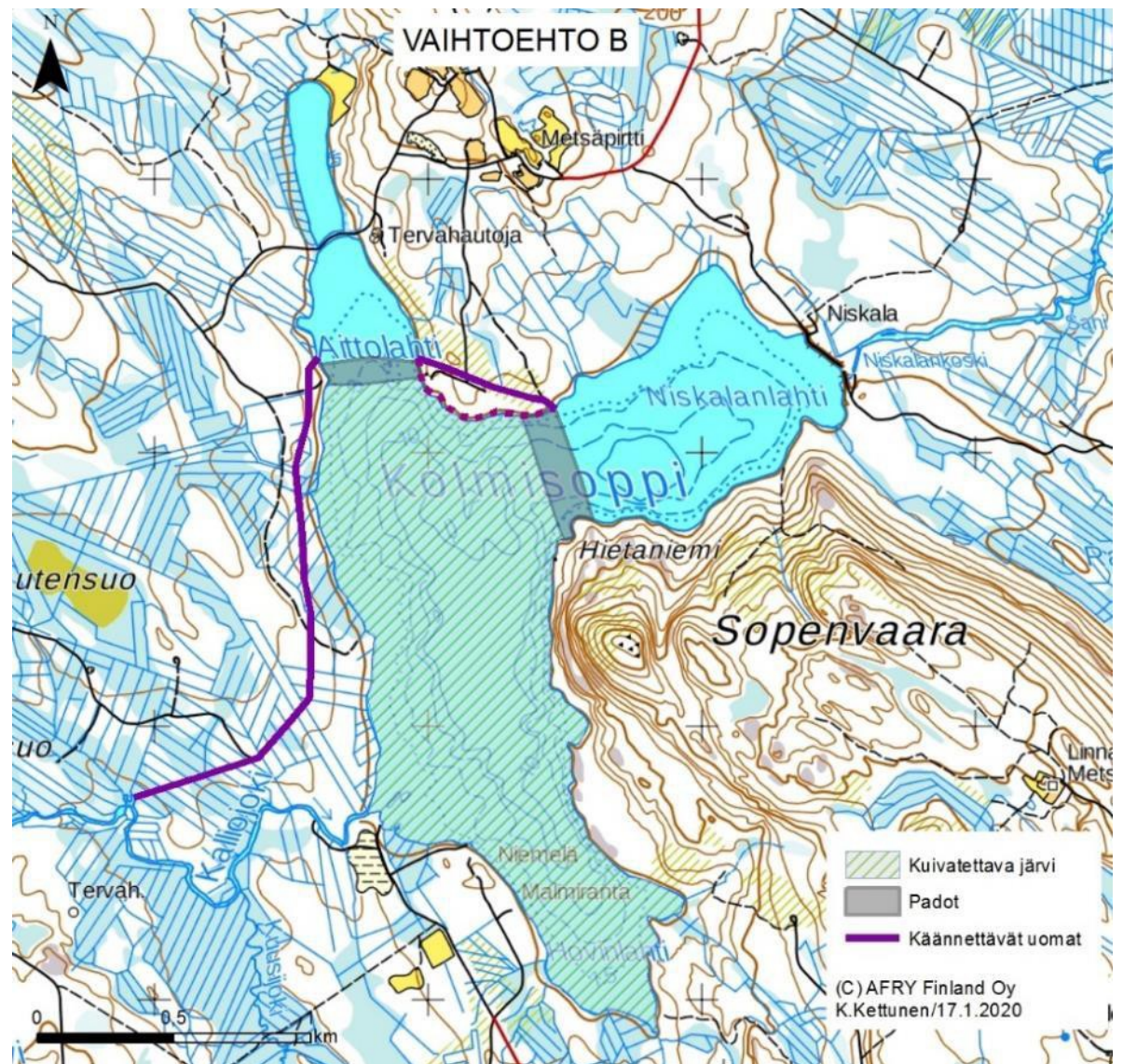
Kuva 2. VE1b ja VE2b patoaminen Niskalanlahden kohdalta. (Pöry Finland Oy 2019)
