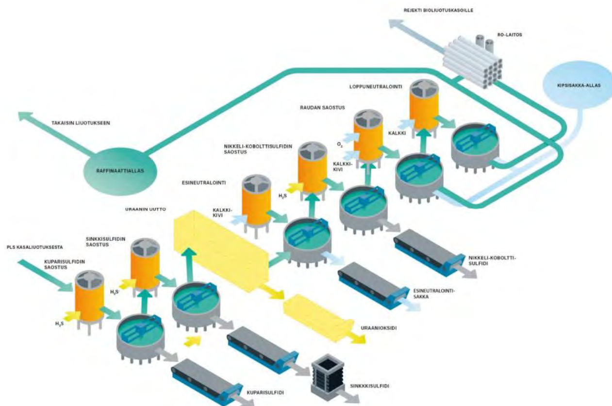
Kuva 3-3. Metallien talteenotto.
