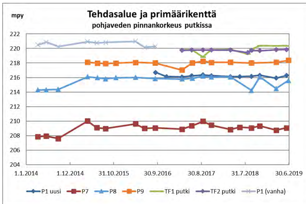
Kuva 4-10 Tehdasalueen ja primäärikentän alueen pohjaveden vedenpinnan korkeus pohjavesiputkissa.
