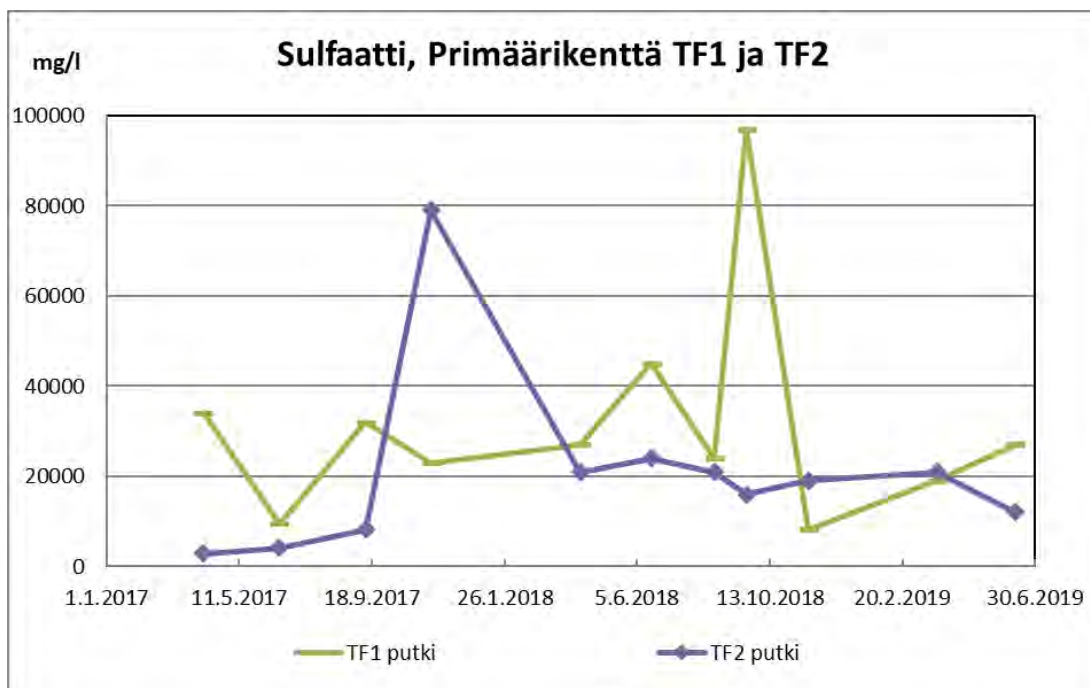
Kuva 4-16 Sulfaattipitoisuus primäärikentän keskikaistan putkissa TF1 ja TF2.
