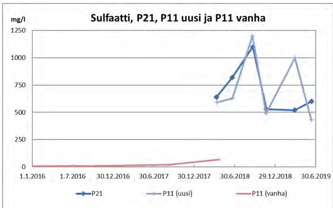
Kuva 4-8 Sivukivialue KL2:n sulfaattipitoisuus pohjavesiputkissa P11 ja P21.
