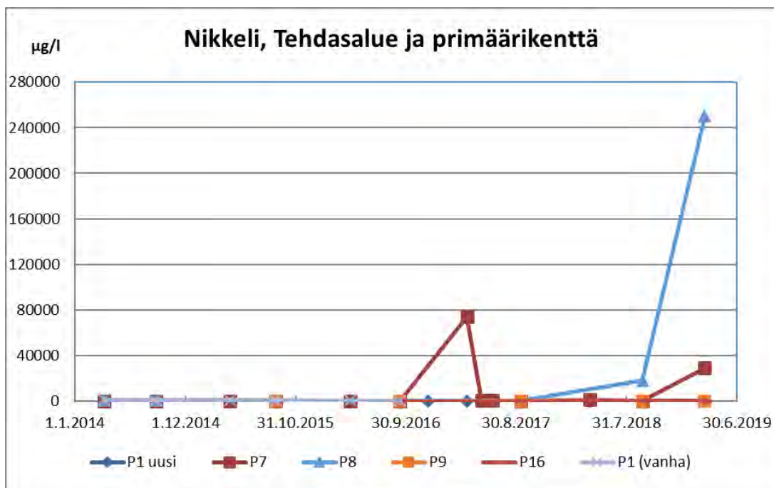
Kuva 4-12 Nikkelipitoisuudet tehdasalueen ja primäärikentän pohjaveden tarkkailupisteissä.
