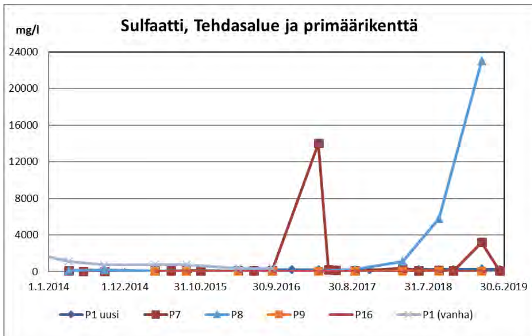
Kuva 4-15 Sulfaattipitoisuus tehdasalueen ja primäärikentän alueen pohjavesissä.
