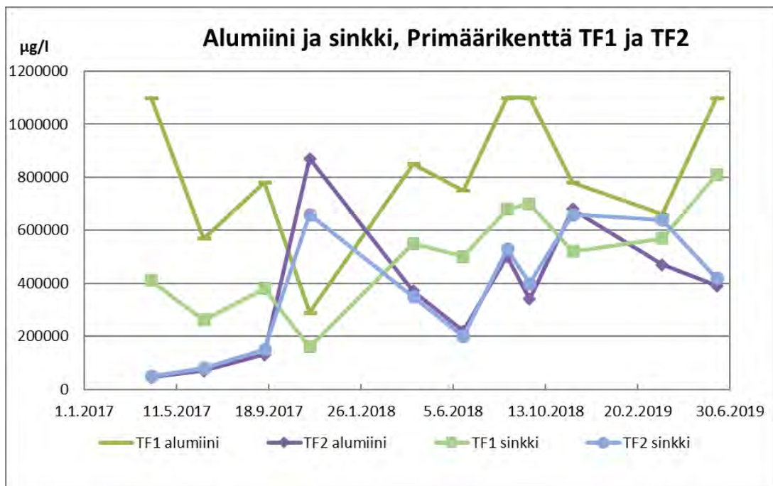
Kuva 4-14 Alumiini- ja sinkkipitoisuudet primäärkentän keskikaistan putkissa TF1 ja TF2
