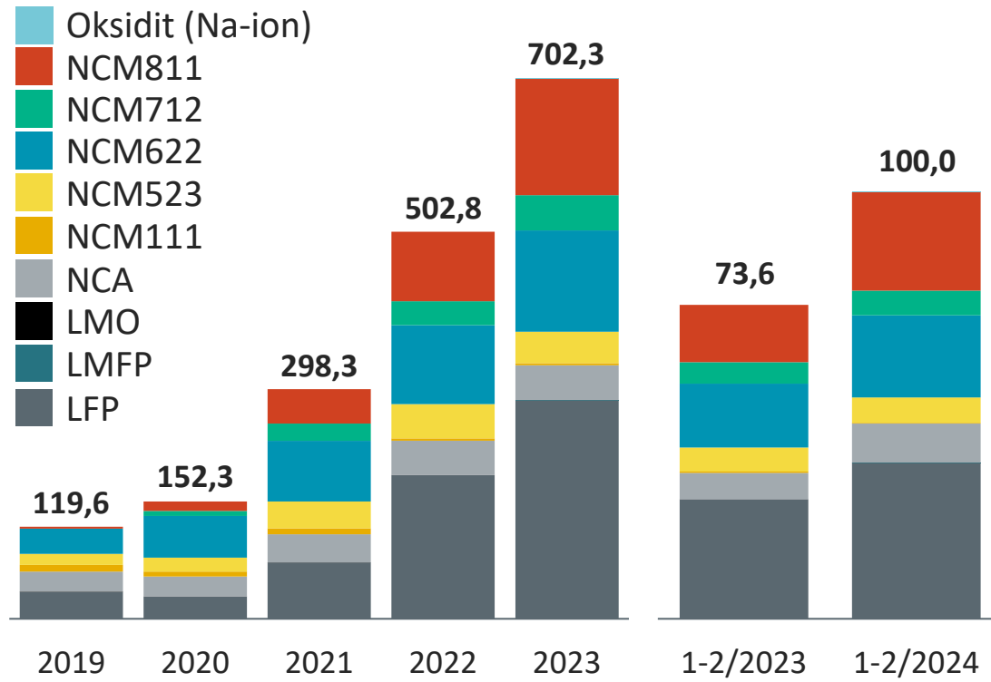
Sähköautojen akkujen katodikemia, GWh
