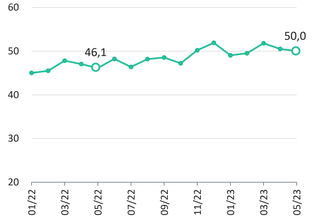
Sähköautojen akkujen myyntipainotettu keskikoko, kWh
