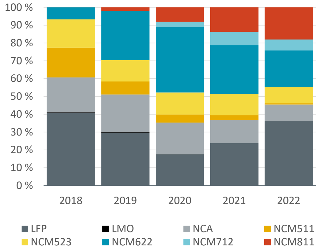
Keskimääräinen sähköautojen akkukemia
