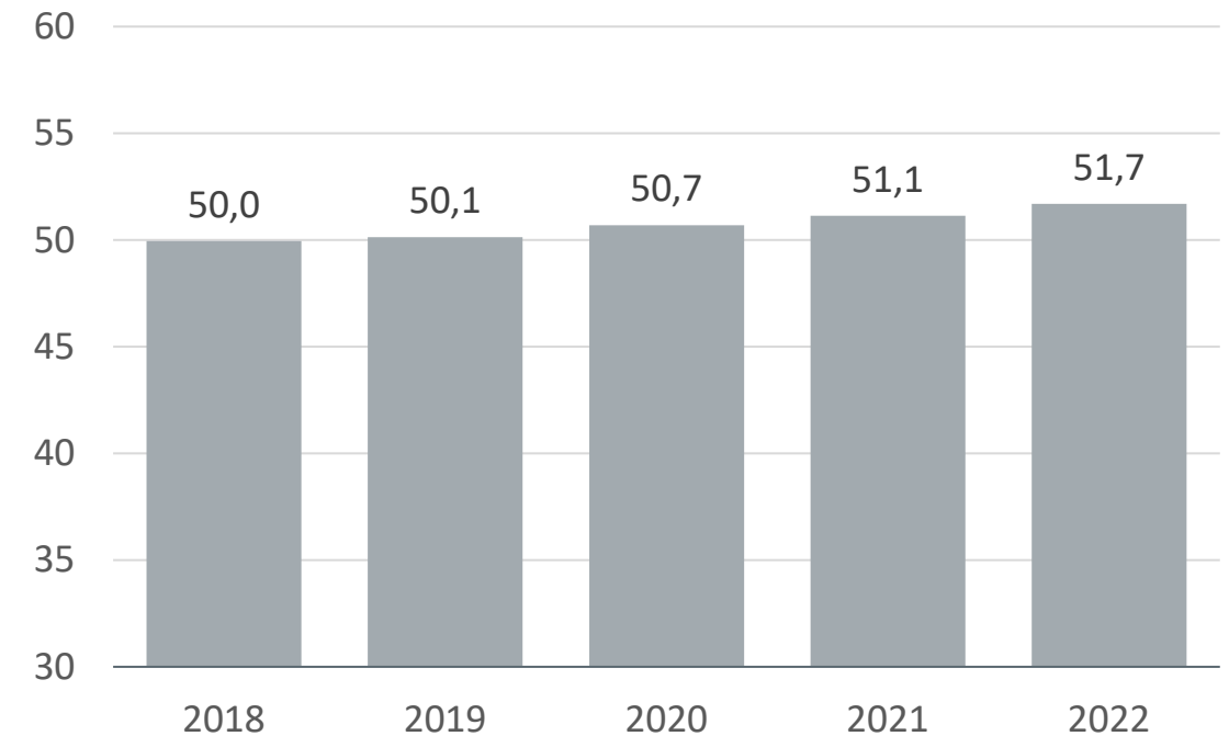
Sähköautojen akkujen myyntipainotettu kesikoko, kWh
