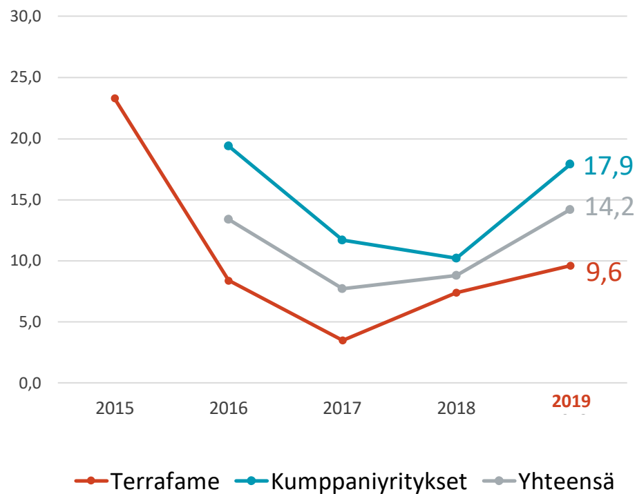
Liukuva 12 kk tapaturmataajuus (LTIFR)
