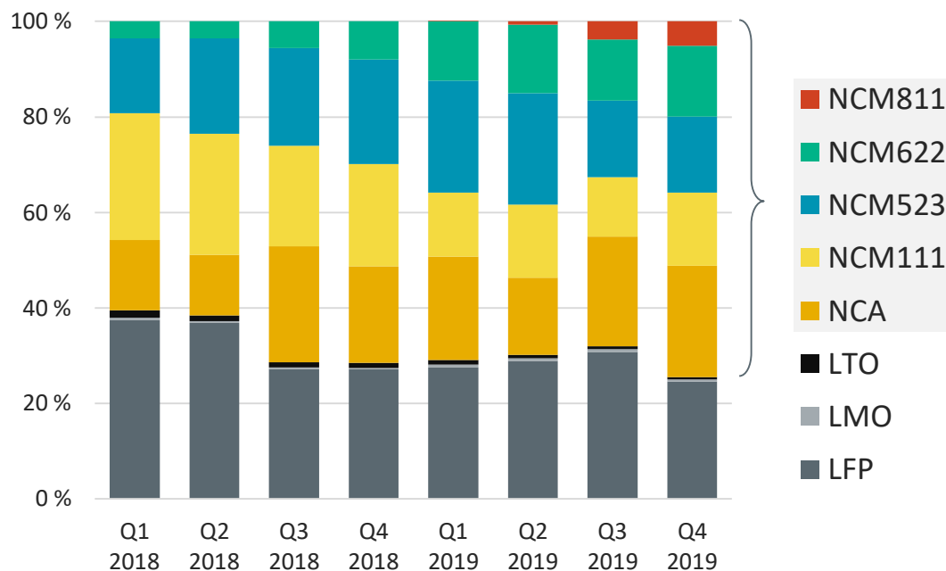
Sähköautojen akkukemia
