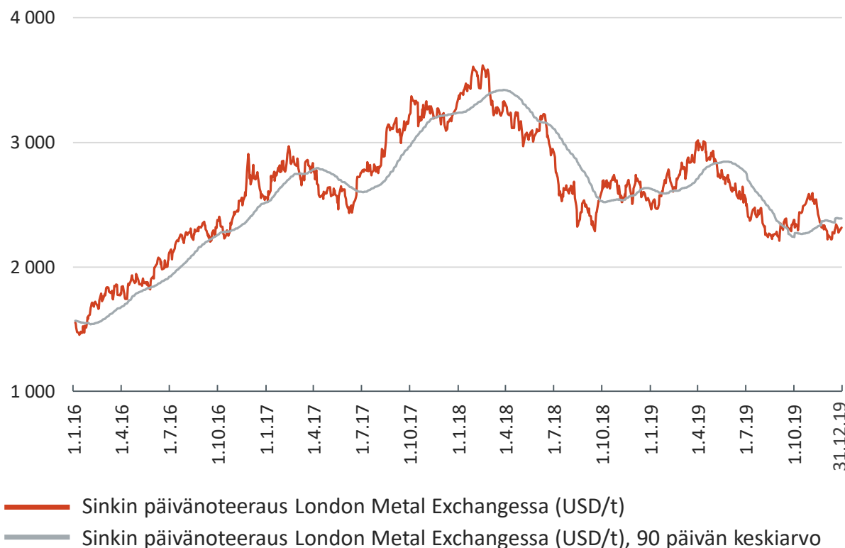
Sinkin hintakehitys (USD/t) 1.1.2016–31.12.2019
